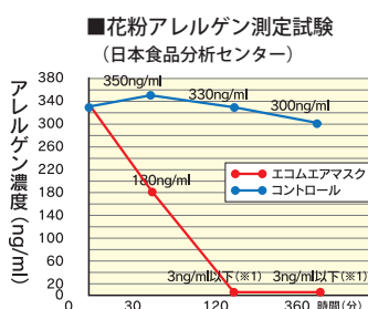
【二酸化塩素の効果試験結果グラフ】
